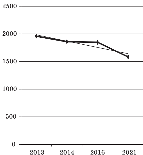
Рис. 1. Линия тренда и кривая количества зарегистрированных НКО на территории Курской области за период с 2013 по 2021 год
