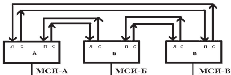
Рис. 2. Схема системы комплексирования комплектов одной ячейки
