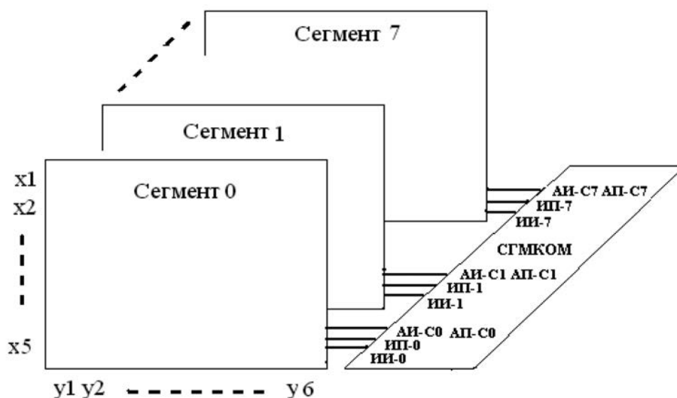
Рис. 5. Структура одного сегмента при организации матрицы 6×5
