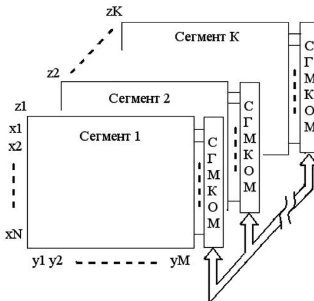
Рис. 4. Структурная схема комплексирования сегментов ВС
