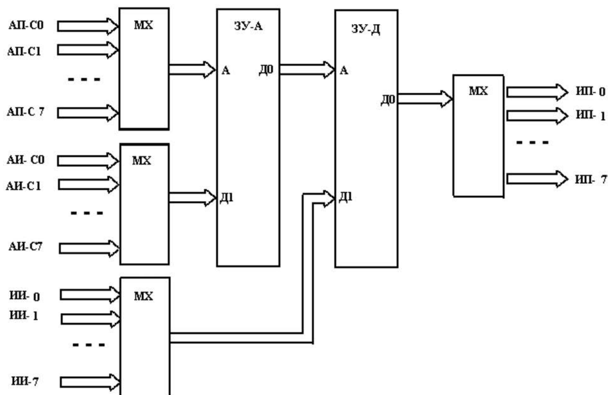
Рис. 6. Структурная схема организации потоков СГМКМ рассматриваемой ВС
